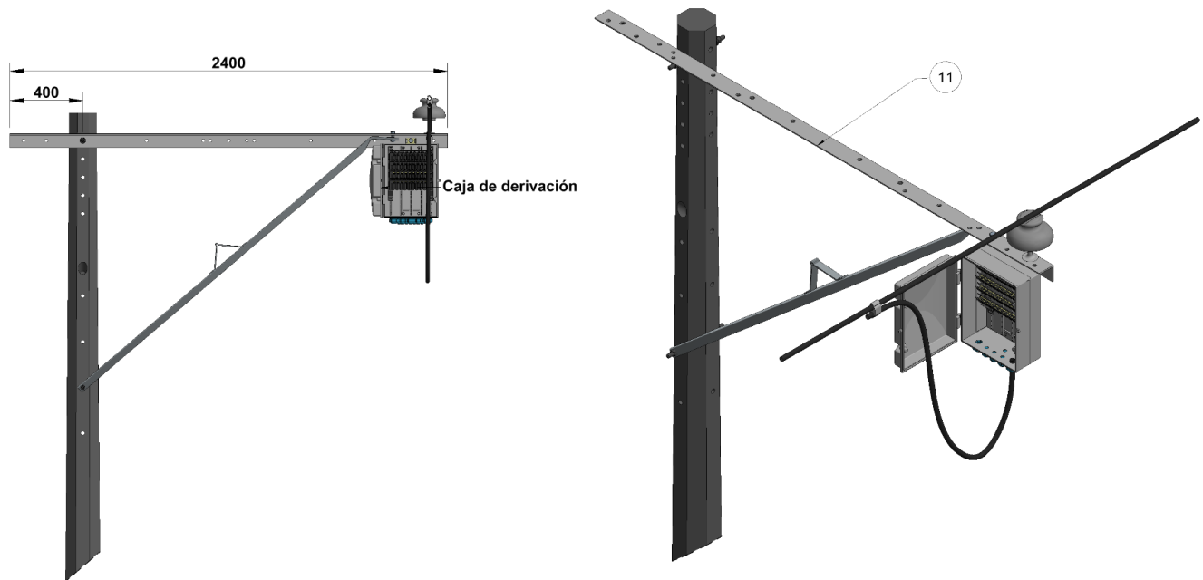
Figura 2. Derivación desde red aérea con caja de derivaciones en cruceta.
