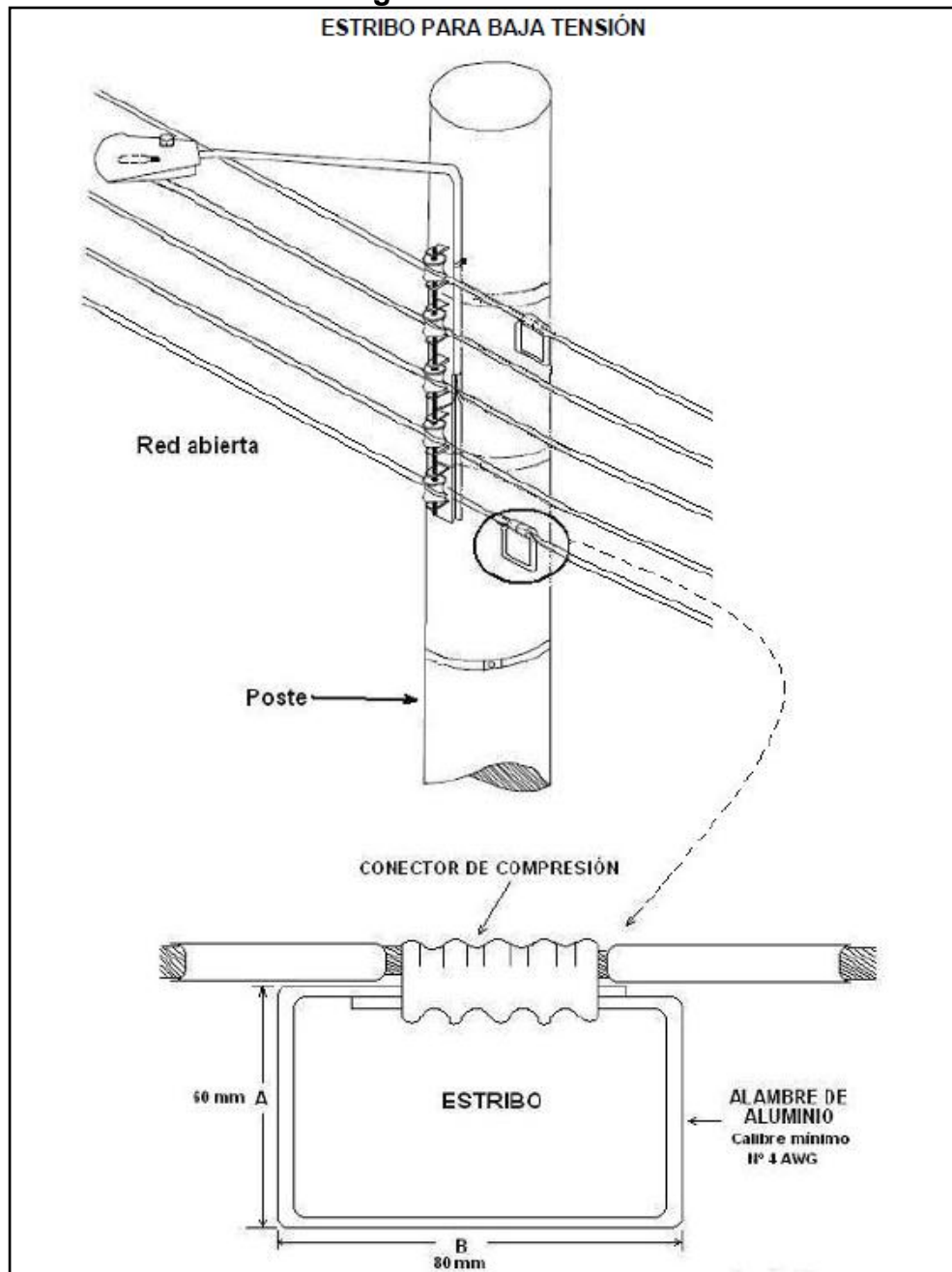
Figura 15. Estribos.
