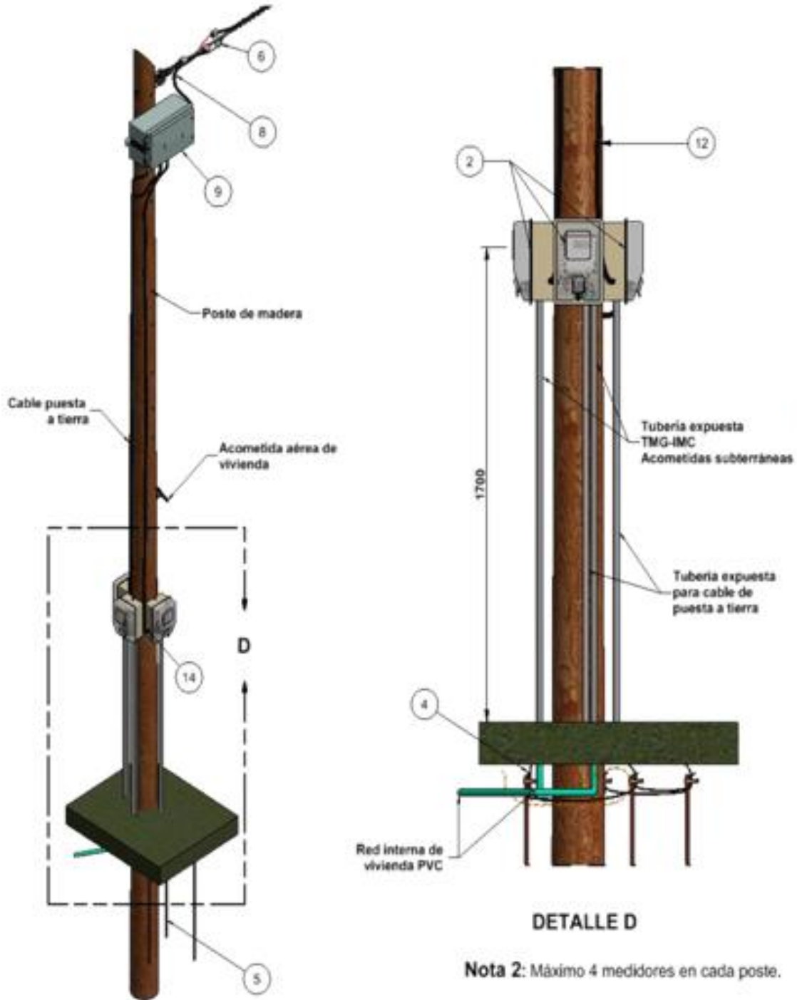
Figura 11. Instalación de medidores de energía en poste.
