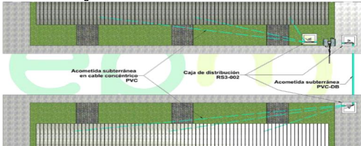
Figura 5. Acometida canalizada o subterránea.
